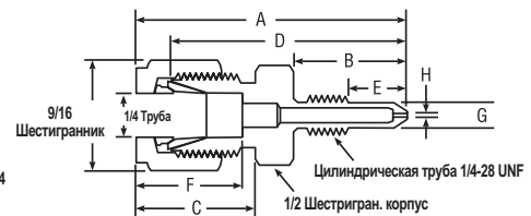
Переходник для калибровки датчиков перепада давления Honeywell
